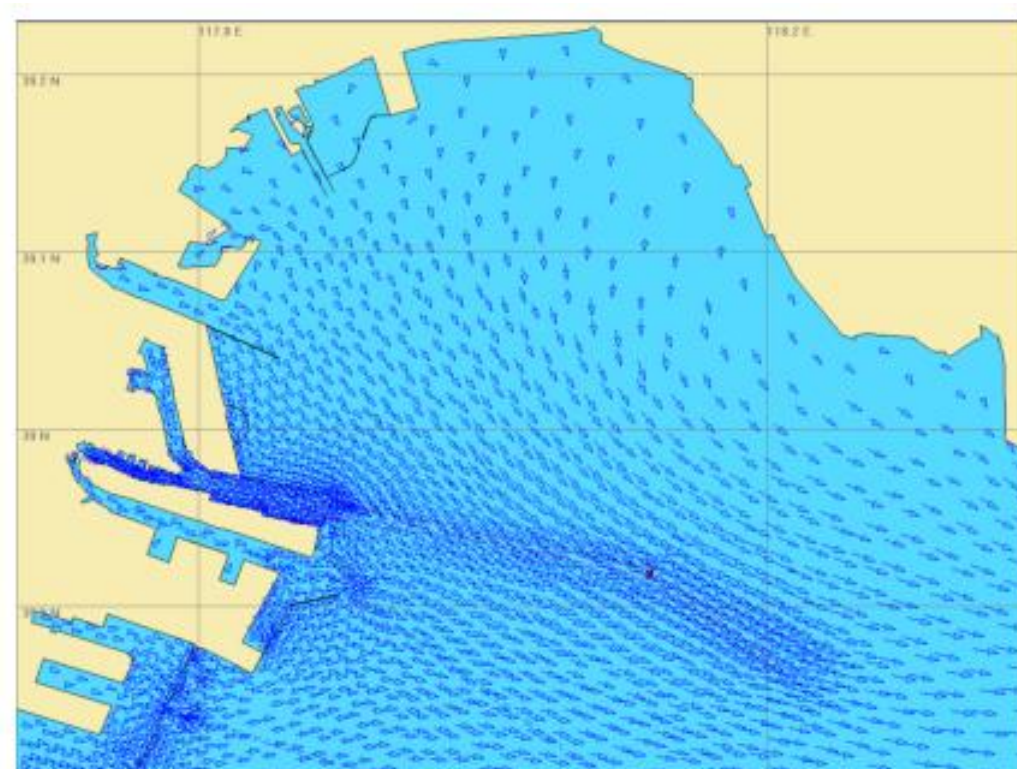
图 4-3-4 大范围潮流场（涨潮阶段）示意图
