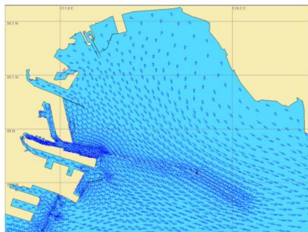
图 4-3-5 大范围潮流场（落潮阶段）示意图
