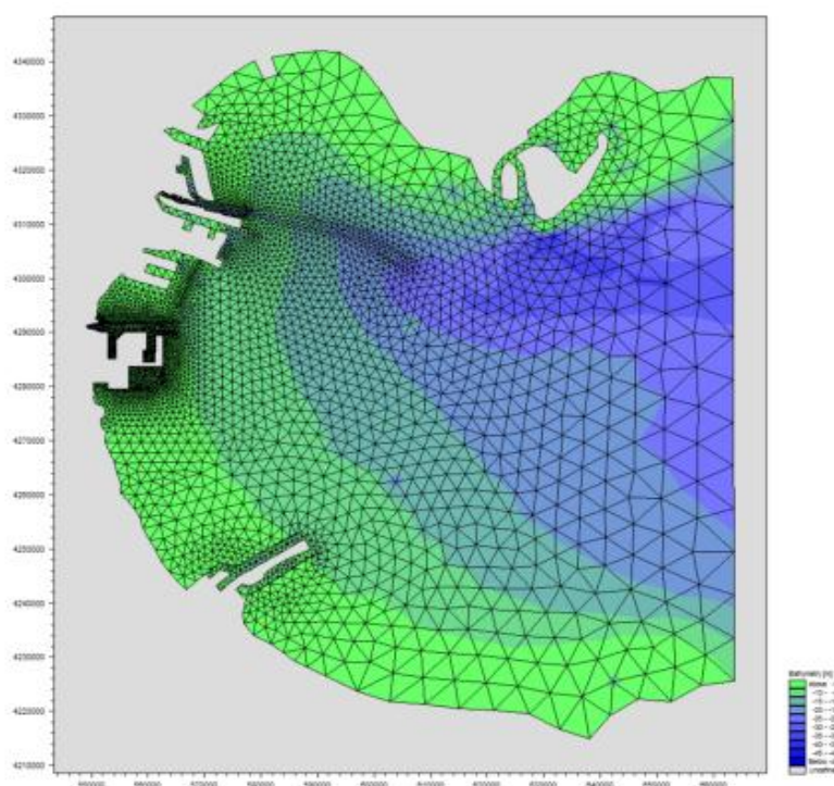
图 4-3-3 计算范围及网格剖分示意图
