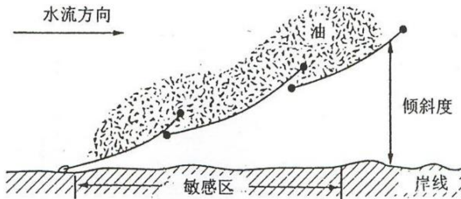
图 4-2 围油栏转移
